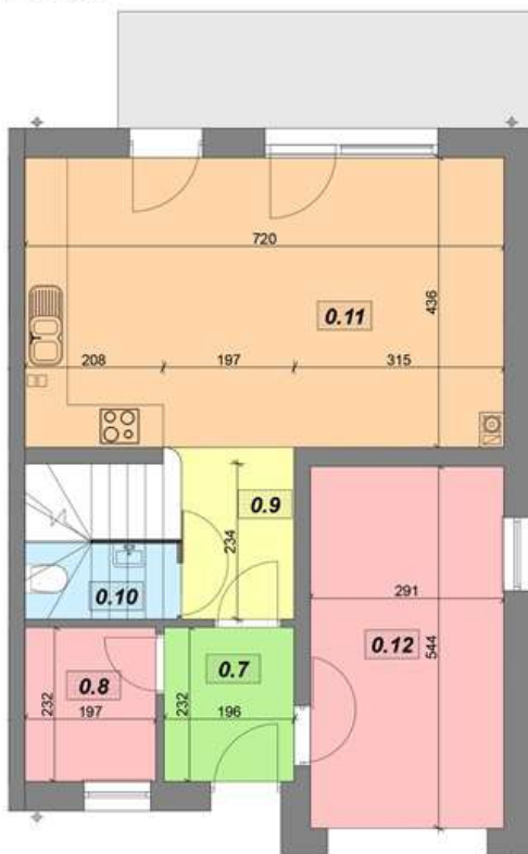
Powierzchnia parteru lokal L3
